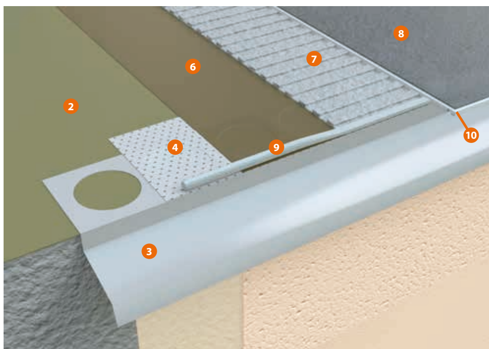
obr. 1/b – Detail osazení balkonového profilu s vloženým vyplňovacím PE provazcem pod přesahem dlažby tvořící okapový nos
